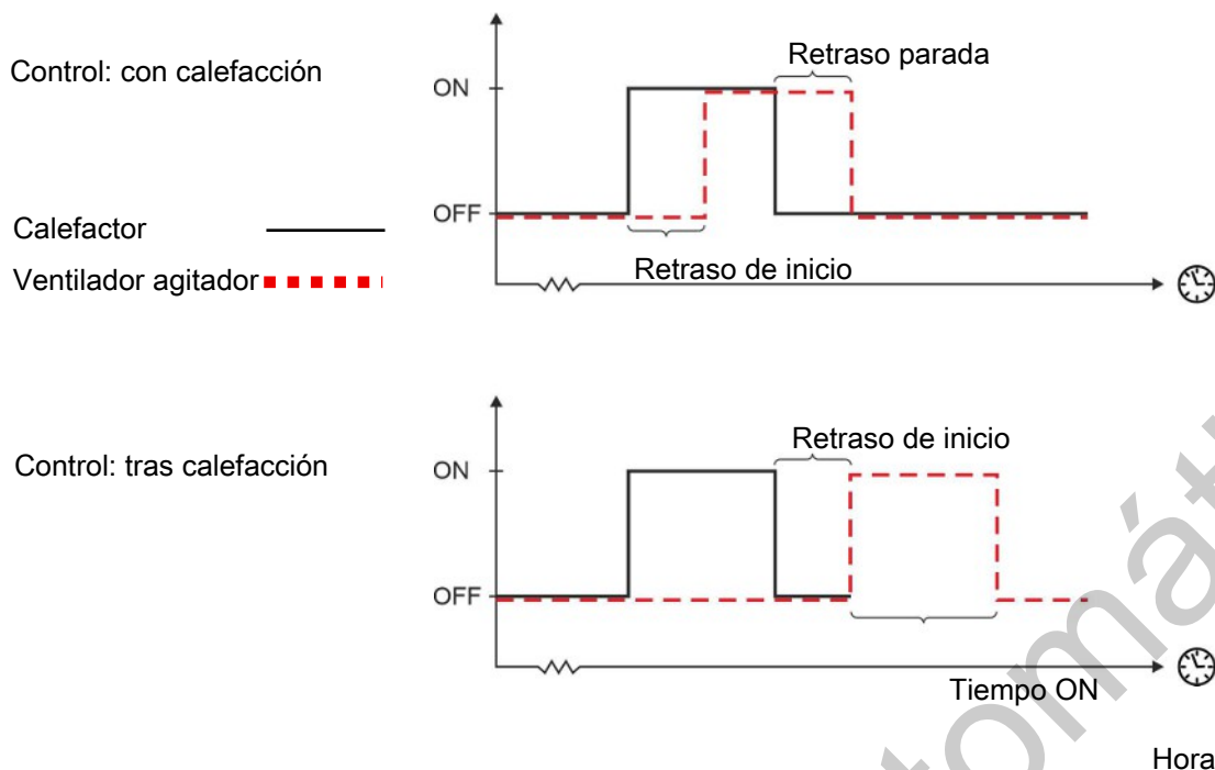
Figura 25: Control con calefacción
