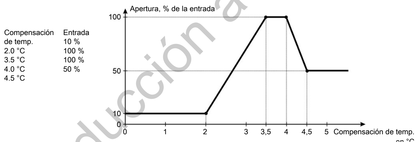
Figura 10: Entrada Combi difusa: apertura continua reducida con una temperatura exterior alta
