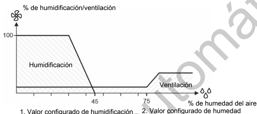
Figura 12: 1. Disminuir la humedad del aire. La humedad del aire está por debajo del valor configurado de humidificación. El controlador inicia la humidificación. 2. Incrementar la humedad del aire. La humedad del aire está por encima del valor configurado de humedad. El controlador aumenta la ventilación.
