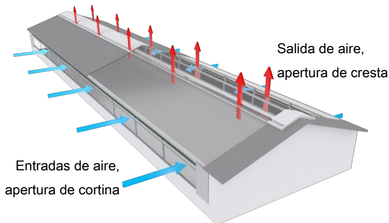
Figura 19: Por ejemplo, una nave con ventilación natural pura, con aperturas de cortina en los laterales y una apertura de cresta en el techo.
