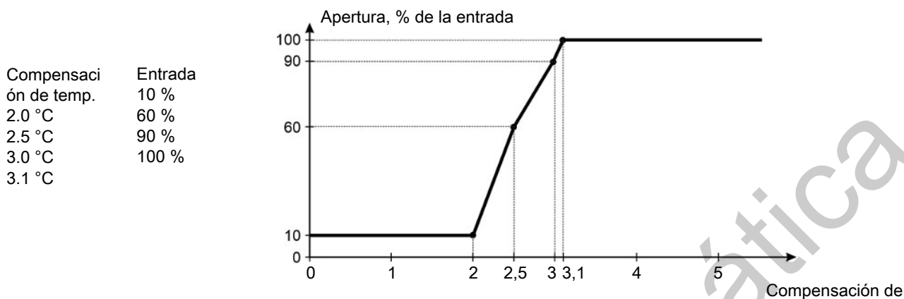
Figura 11: entrada Combi difusa. Apertura continua basada en la temperatura interior y exterior
