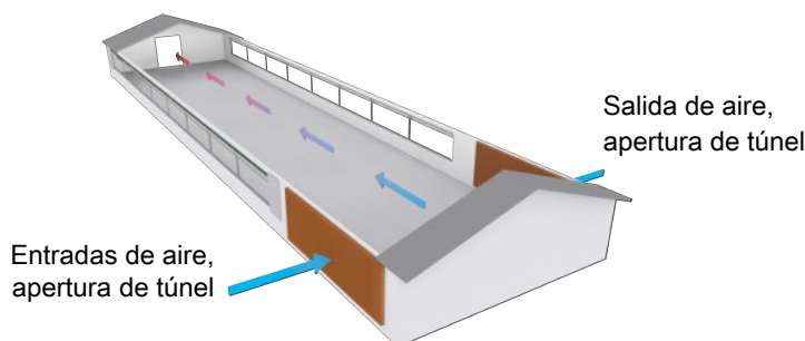
Figura 21: Ejemplo de nave ganadera con ventilación natural en combinación con ventilación túnel, ventilación túnel.
