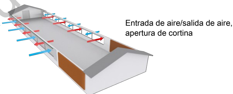
Figura 20: Ejemplo de una nave ganadera con ventilación natural en combinación con ventilación de túnel, ventilación natural.
