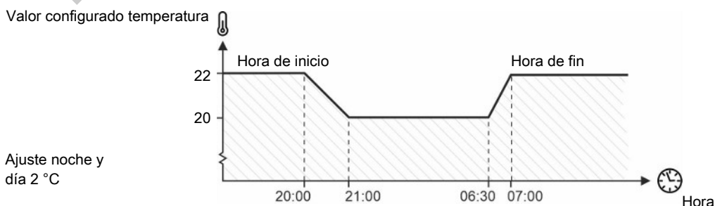
Figura 7: Ajuste de día y noche establecido como un descenso nocturno de la temperatura.
