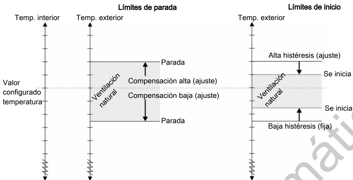
Figura 22: Iniciar y detener en relación con la temperatura exterior. Los límites de temperatura se establecen como compensados con el valor configurado de temperatura.
