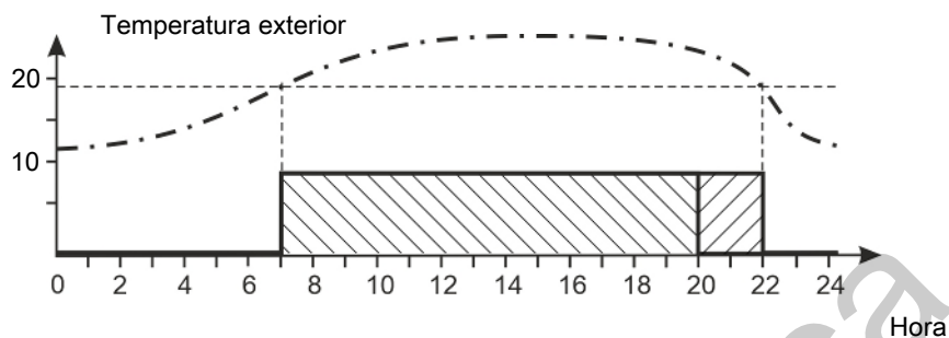
Figura 32: Pulverización según la hora y la temperatura exterior
