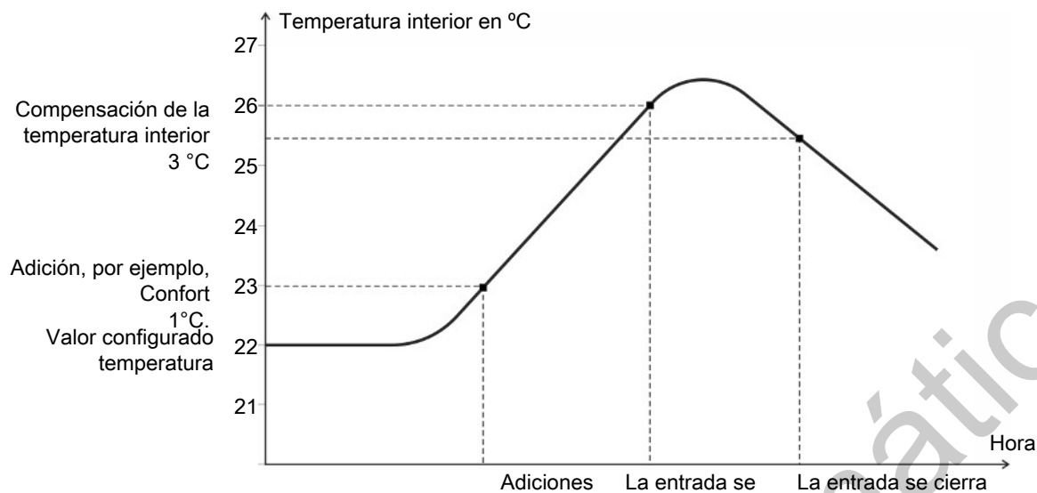
Figura 9: Entrada Combi difusa: temperatura interior regulada
