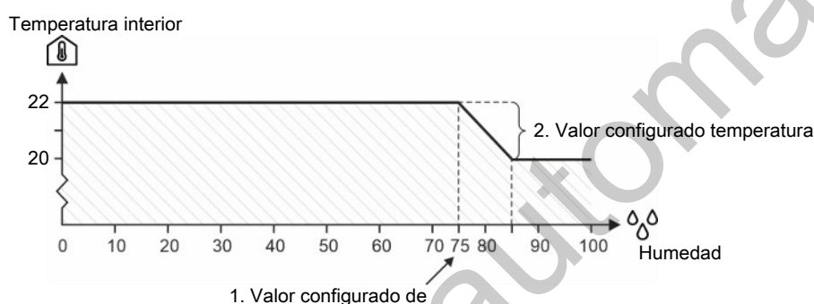
Figura 15: Control de humedad con reducción de temperatura
