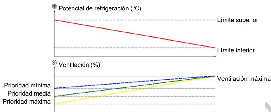
Figura 28: Cuanto mayor sea el potencial de refrigeración, mayor será la prioridad del inicio de refrigeración temprana.
