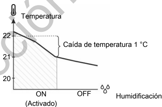
Figura 13: Disminuir la temperatura: La humidificación se desconectará si la temperatura interior está 1 °C por debajo del Valor configurado de temperatura. De lo contrario, la humidificación podría hacer que la temperatura interior descendiera aún más.
