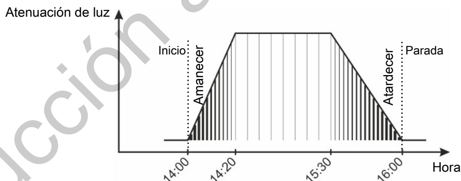
Figura 39: Atenuación de luz normal El amanecer y el atardecer se integran en el período de luz.
