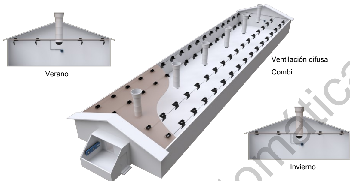
Figura 8: Combi-difusa combina las mejores propiedades de dos sistemas de ventilación: Difuso y LPV.
